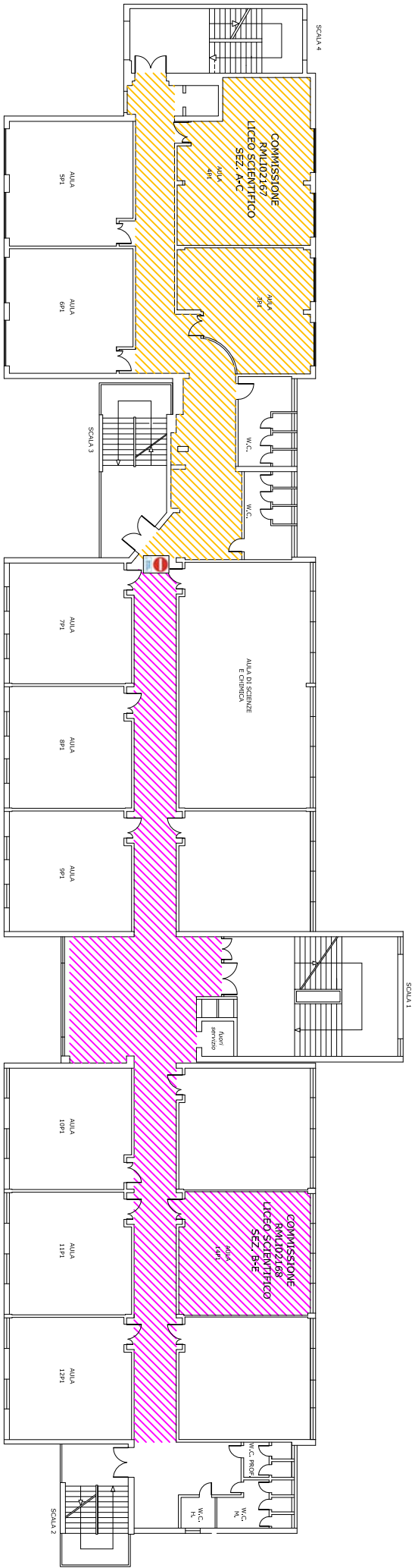
PRIMO PIANO
